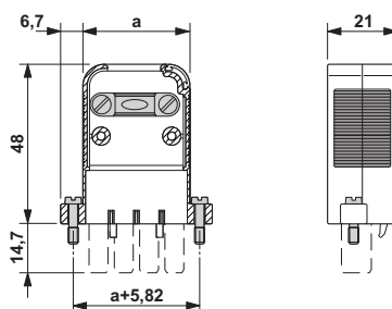
Rysunek wymiarowy
