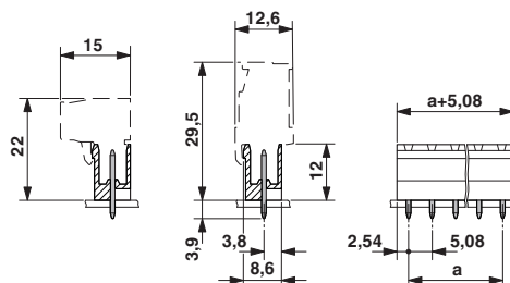
Rysunek wymiarowy
