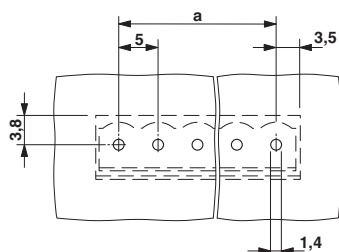
Szablon wierceń
