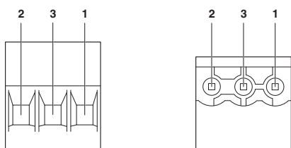
rysunek schematyczny
