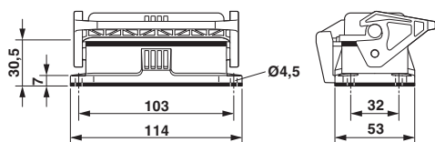
Rysunek wymiarowy
