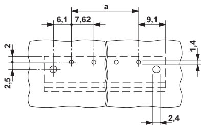
Szablon wierceń
