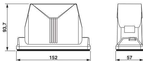
Rysunek wymiarowy
