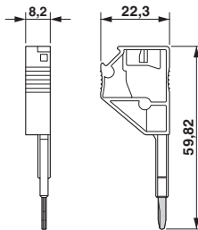
Rysunek wymiarowy
