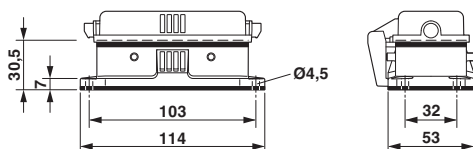
Rysunek wymiarowy
