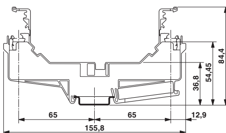
Rysunek wymiarowy
