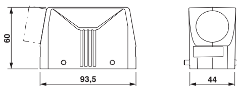
Rysunek wymiarowy
