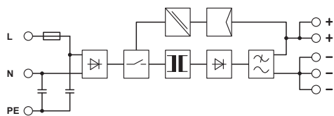
Schemat blokowy
