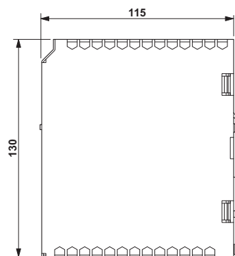
Rysunek wymiarowy
