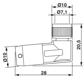
Rysunek wymiarowy
