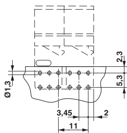
Szablon wierceń
