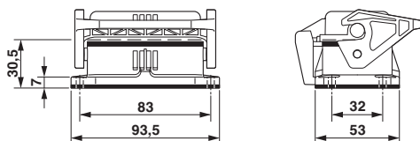
Rysunek wymiarowy
