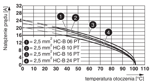
Krzywa redukcyjna
