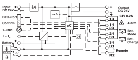
Schemat blokowy
