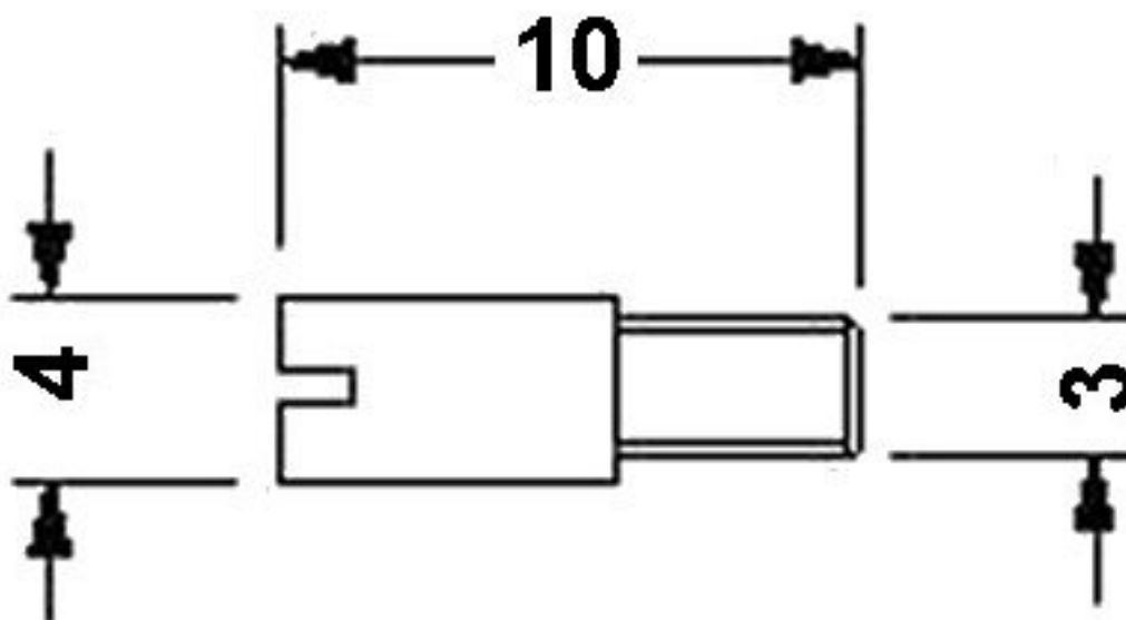
Rysunek wymiarowy
