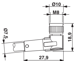
Rysunek wymiarowy
