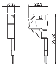
Rysunek wymiarowy
