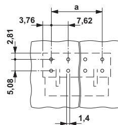
Szablon wierceń
