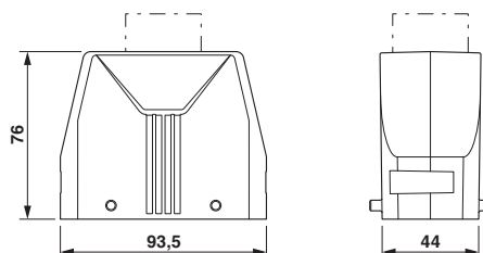
Rysunek wymiarowy
