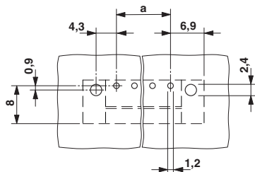
Szablon wierceń
