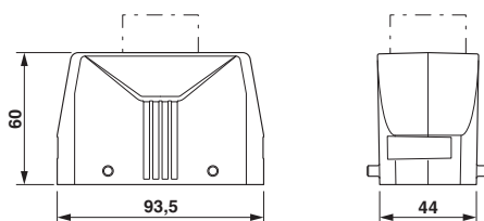
Rysunek wymiarowy
