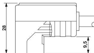
wtyk zaworowy, konstrukcja C, z boku
