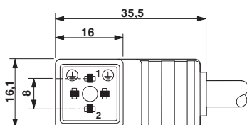
Wtyk zaworowy, typ C
