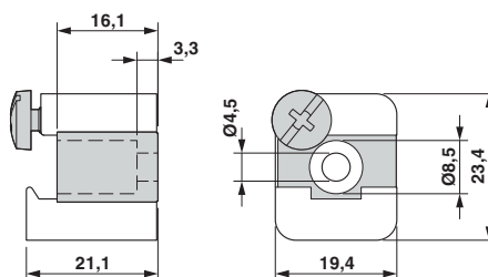
Rysunek wymiarowy
