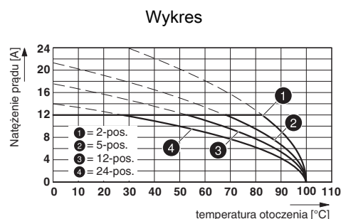
Typ: ICV 2,5/...-G-5,08 z MSTBA 2,5/...-G-5,08
