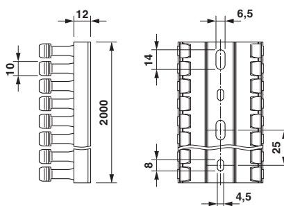
Rysunek wymiarowy
