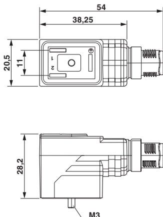
Rysunek wymiarowy
