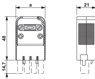
Rysunek wymiarowy
