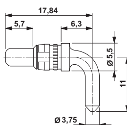
Rysunek wymiarowy
