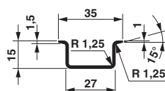
Rysunek wymiarowy
