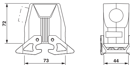
Rysunek wymiarowy
