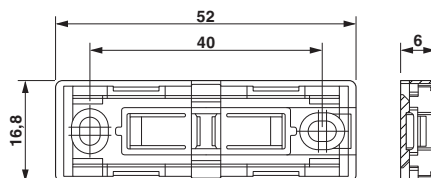
Rysunek wymiarowy
