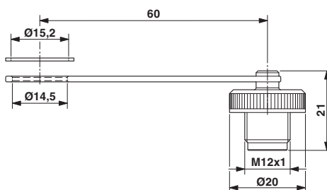
Rysunek wymiarowy
