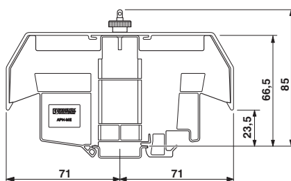
Rysunek wymiarowy
