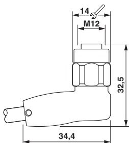
Rysunek wymiarowy
