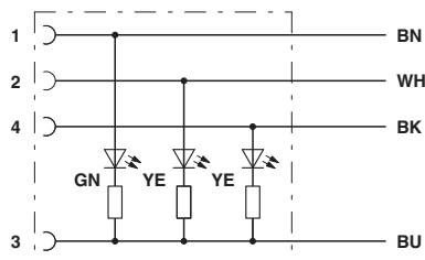
Przyporządkowanie styków wtyków M12 i gniazd M12
