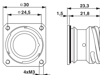
Rysunek wymiarowy
