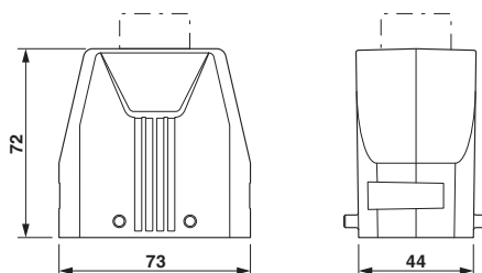
Rysunek wymiarowy
