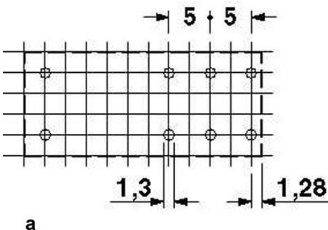
Szablon wierceń
