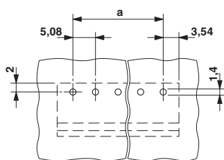
Szablon wierceń
