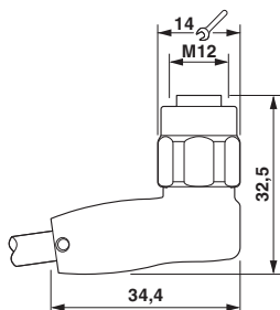
Rysunek wymiarowy
