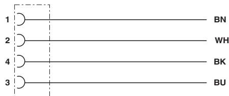
Przyporządkowanie styków wtyków M12 i gniazd M12
