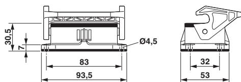
Rysunek wymiarowy
