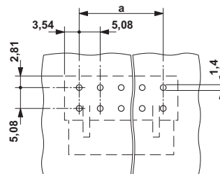
Szablon wierceń
