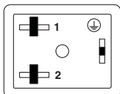
Układ styków wtyk zaworowy, typ BI
