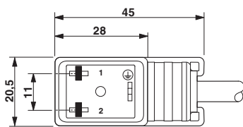
Wtyk zaworowy typ BI
