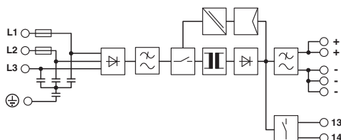
Schemat blokowy
