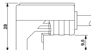
Rysunek wymiarowy
