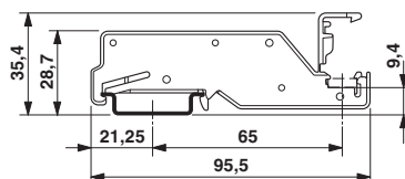
Rysunek wymiarowy
