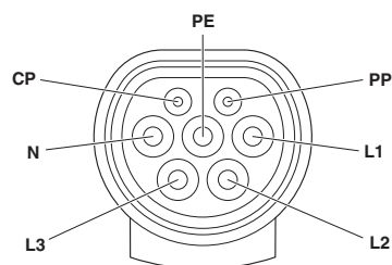
Przyporządkowanie pinów wtyki do ładowania do pojazdów
