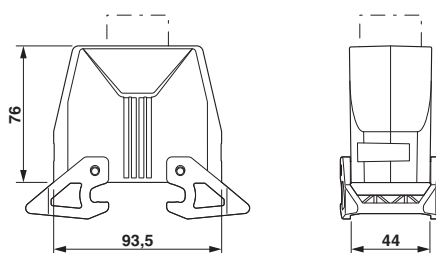
Rysunek wymiarowy
